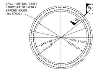
3 DETAIL: TEMPLATE RING SCALE: 1:4
